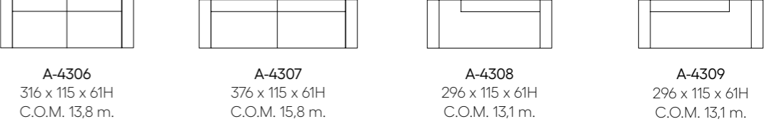
A-4300 130 x 115 x 61H C.O.M. 4,5 m. A-4301 160 x 115 x 61H C.O.M. 5,4 m. A-4302 210 x 115 x 61H C.O.M. 6,9 m. A-4303 186 x 115 x 61H C.O.M. 9,3 m. A-4304 216 x 115 x 61H C.O.M. 10,2 m. A-4305 266 x 115 x 61H C.O.M. 12,3 m.
