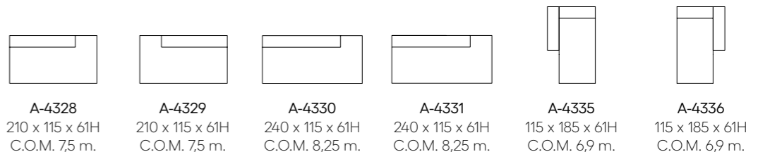
A-4322 238 x 115 x 61H C.O.M. 9,9 m. A-4323 238 x 115 x 61H C.O.M. 9,9 m. A-4324 268 x 115 x 61H C.O.M. 10,7 m. A-4325 268 x 115 x 61H C.O.M. 10,7 m. A-4326 160 x 115 x 61H C.O.M. 5,4 m. A-4327 160 x 115 x 61H C.O.M. 5,4 m.
