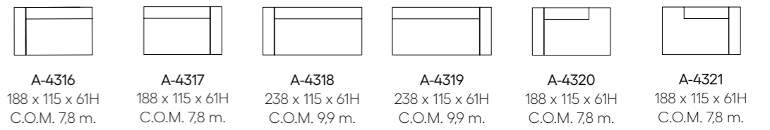
A-4310 188 x 115 x 61H C.O.M. 7,8 m. A-4311 188 x 115 x 61H C.O.M. 7,8 m. A-4312 268 x 115 x 61H C.O.M. 10,7 m. A-4313 268 x 115 x 61H C.O.M. 10,7 m. A-4314 158 x 115 x 61H C.O.M. 6,9 m. A-4315 158 x 115 x 61H C.O.M. 6,9 m.
